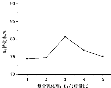
图4 复合乳化剂 SDS 和 OP - 10 的总量对 D_4 转化率的影响
