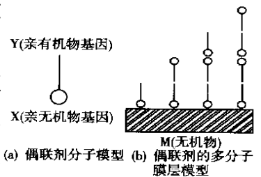
图 2 无机材料表面上偶联剂分子的排列简图
