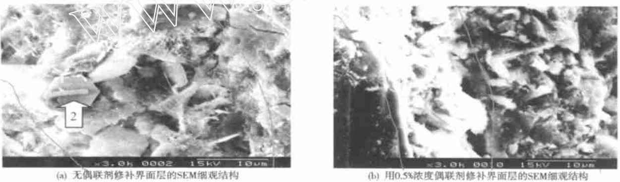
图 3 花岗石-砂浆界面层微结构
