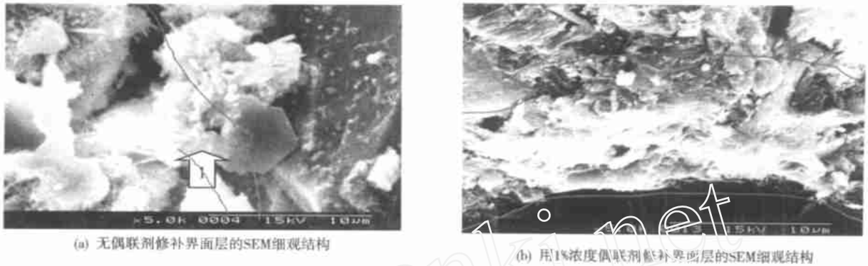
图 3 花岗石-砂浆界面层微结构
